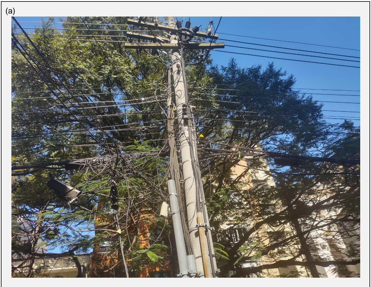
Figura 3 - Fotos do compartilhamento da infraestrutura da CEEE-D Equatorial na município de Porto Alegre, Rua Henrique Dias.
