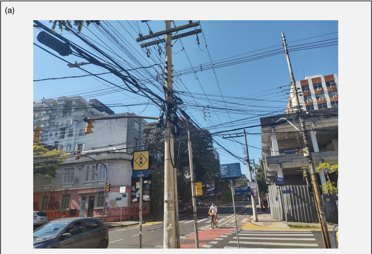
Figura 1 – Fotos do compartilhamento da infraestrutura da CEEE-D Equatorial no município de Porto Alegre, Rua Felipe Camarão.
